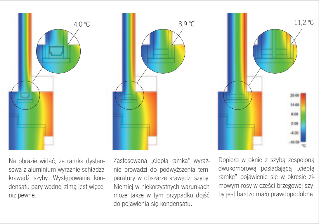
Obrazy termowizyjne przekroju okna drewnianego z szybą zespoloną jedno- i dwukomorową. Temperatura w pomieszczeniu +20 °C, temperatura na zewnątrz -10 °C
